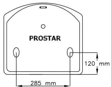
VYN OVANIFRÅN
